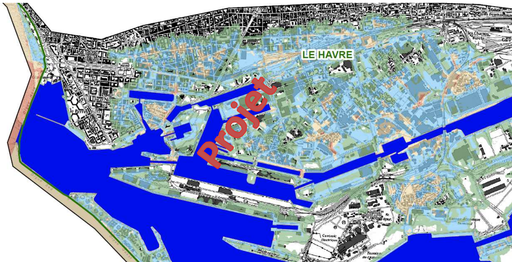
Aléa submersion marine 2100 sur le centre ville du Havre
